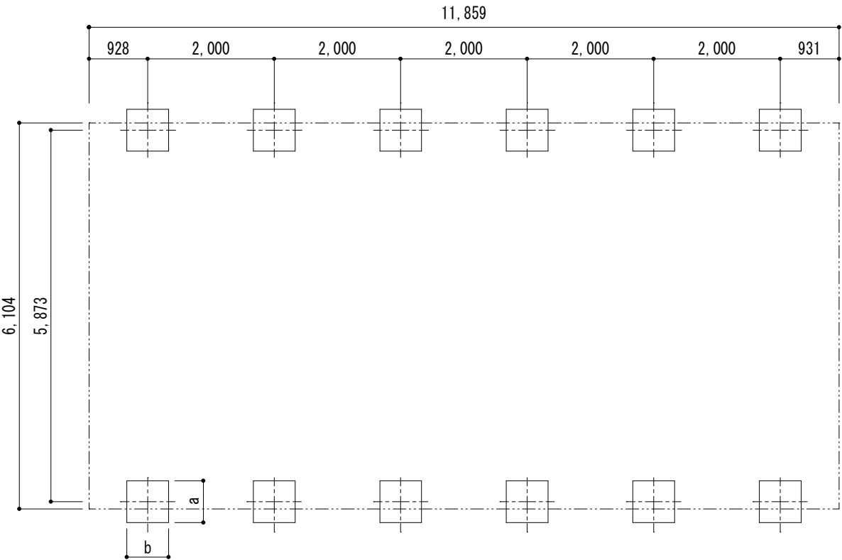
■基礎配置図
